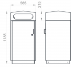
Pyramid Frontry (304SSPF)
