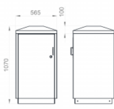
Pyramid Top (304SSPT)
